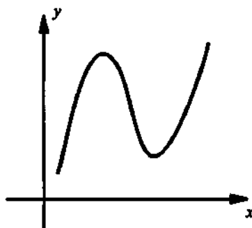
Немонотонная функция
